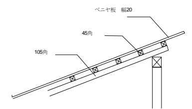
屋根 詳細図
