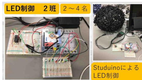
■ “ブロックプログラム:Studuino”によるオブジェ制御
