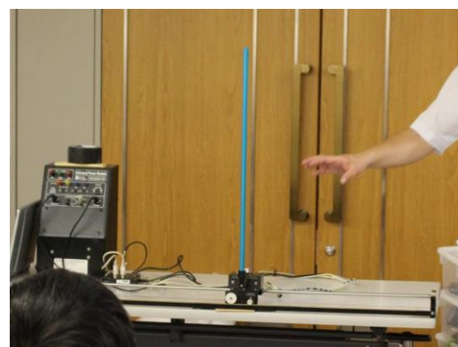
■倒立振りロボットの自動制御
