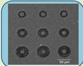
ダイヤモンドライク カーボンのマイクロギヤ
