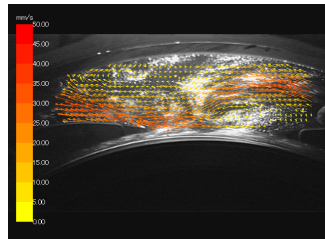
ジャーナル軸受内潤滑流体の流れの可視化例
