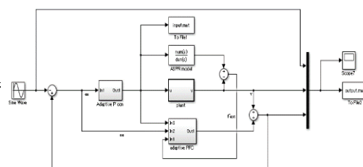
MATLAB/Simulink を利用した適応制御系設計
