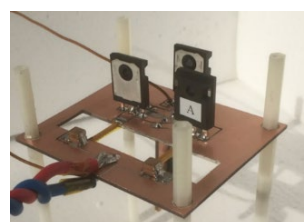
SiC MOSFET の並列回路
