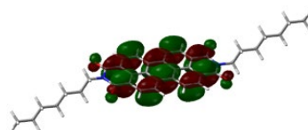
電子状態の第一原理計算
