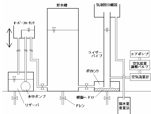
実験装置
